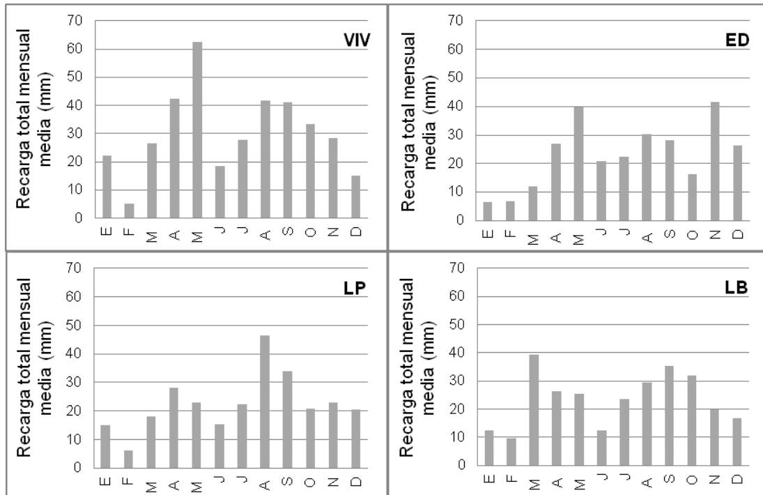
Figura 4. Recarga total media mensual para el período 2007-2014.
