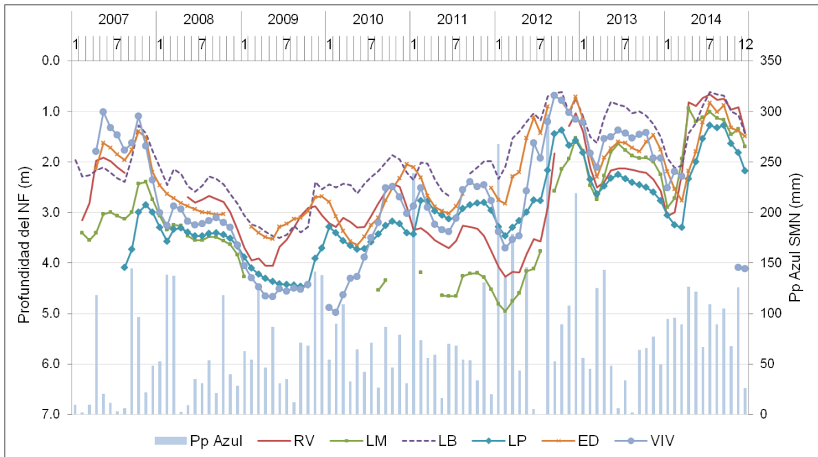
Figura 2. Evolución de la profundidad de los niveles freáticos y de las precipitaciones de la estación Azul SMN durante el período analizado.
