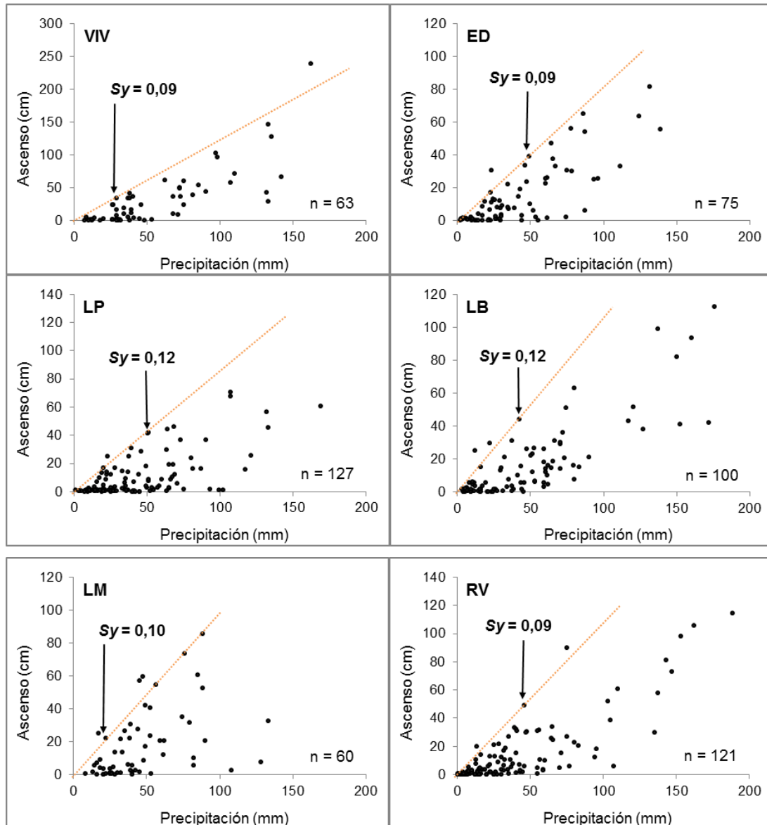
Figura 3. Gráficos para la determinación de Sy.
