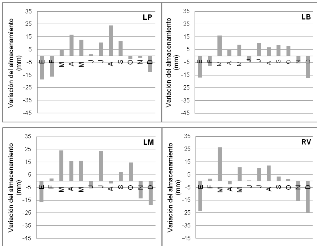
Figura 5 (cont.). Variación del almacenamiento medio mensual para el período 2007-2014, supuesto nulo el escurrimiento superficial.
