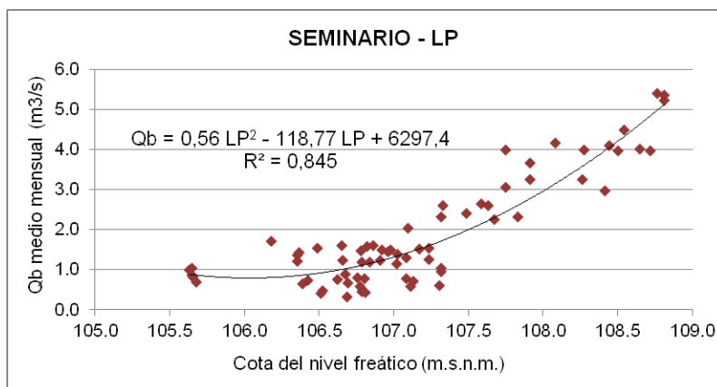
Figura 6. Ajuste obtenido en la estación LP.
