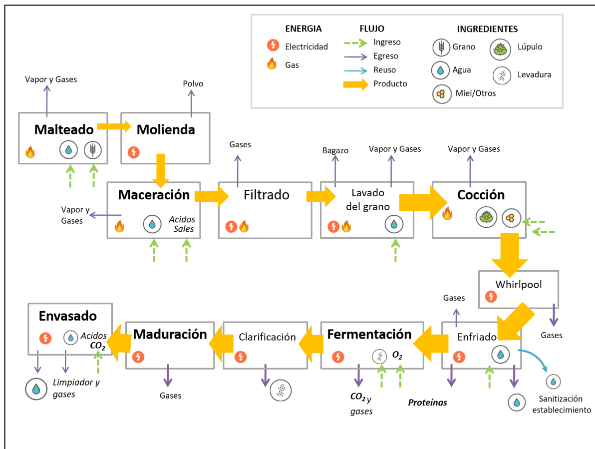
Figura 2. Análisis del ciclo de vida de la cerveza artesanal
